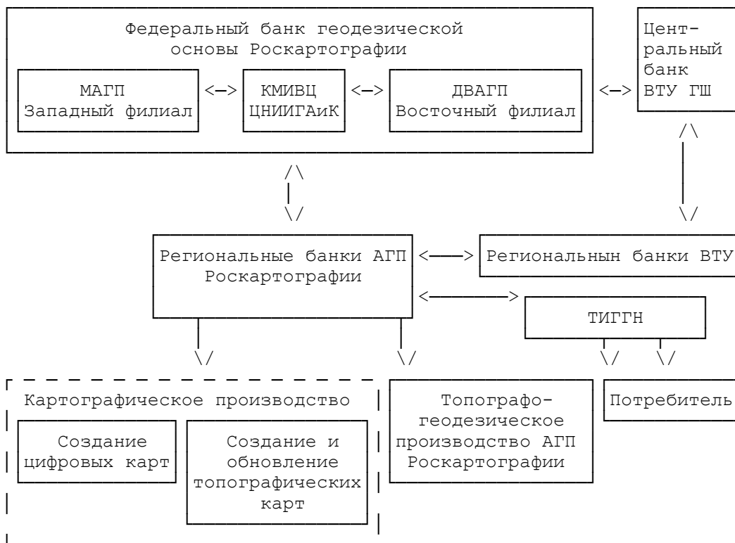
Рис. 5. Структура функционирования банков геодезической основы Роскартографии в системе топографо-геодезического и картографического производства.
